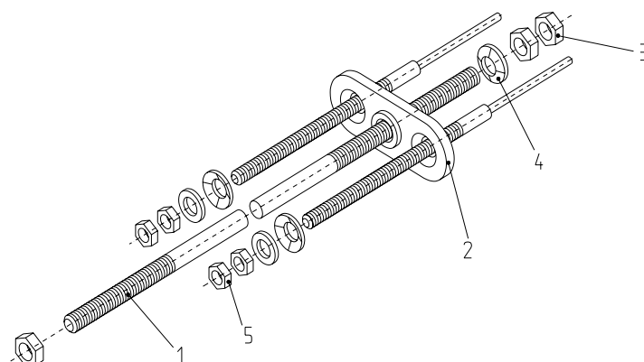
Abb 1. Bremsgestänge
